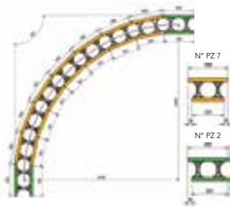
Disposizione curva con raggio 1950 mm Kurvenanordnung mit einem Radius von 1950 mm
