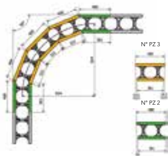
Disposizione curva con raggio 924 mm Kurvenanordnung mit einem Radius von 924 mm
